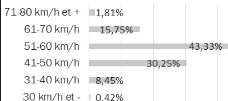
Véhicules sortant du village vers l'ouest - 50 km/h
