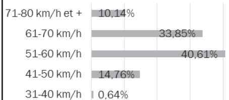
Véhicules se dirigeant vers l'est 60 km/h
