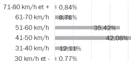
Véhicules entrant dans le village vers l'est - 50 km/h
